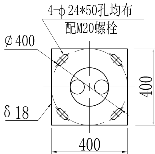
法兰平面示意图
