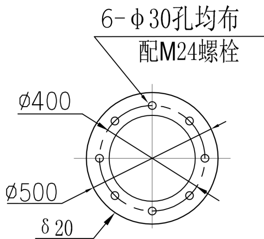
底部法兰平面图
